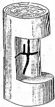
Рис. 16. Обрубок дуба с гнздом непарного корофиды в древесине ( Xyleborus dispar ). В уменьшенном виде.
