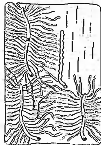
Рис. 10. Кусокъ сосны, съ внутренней поверхностью, съ гнѣздами большаго лубоѣда ( Hylurgus piniperda ). Въ значительно уменьшенномъ видѣ.
