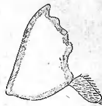
Рис. 4. Верхняя челюсть корофды. Въ значительно увеличенномъ видѣ.
