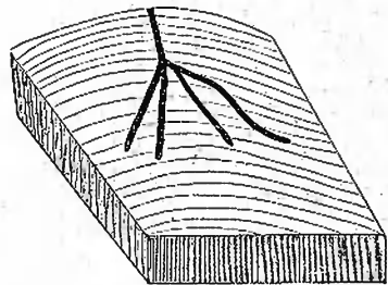
Рис. 19. Гнѣздо полосатаго короѣды въ обрубкѣ ели ( Xyloterus lineatus ). Въ уменьшенномъ видѣ.
