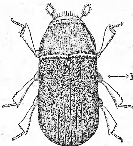
Рис. 3. Корофды ( Polygraphus pubescens ). Въ значительно увеличенномъ видѣ. Черточка справа показывается его натуральную величину.
