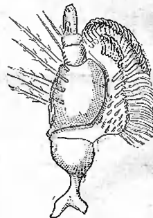
Рис. 5. Нижняя челюсть корофды. Въ значительно увеличенномъ видѣ.
