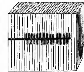
Рис. 20. Обрубокъ ели съ однимъ изъ поперечныхъ ходовъ гнѣзда полосатаго короѣды; видны короткіе вторичные ходы, обитаемые личинками. Въ уменьшенномъ видѣ.
