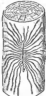
Рис. 2. То же послѣ снятія коры, при чемъ на обнаженной поверхности древесины видны ходы, составляющіе гнѣздо этого заболонника.
