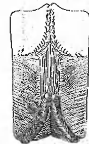
Рис. 9. Одинъ изъ восьми жевательныхъ аппаратовъ, находящихся въ зубу короеда.
