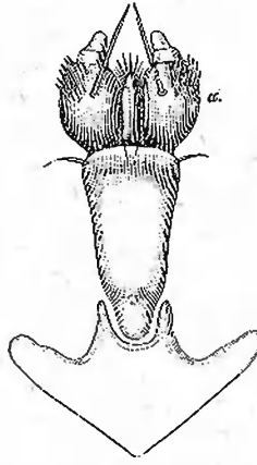
Рис. 7. Нижняя губа корофды: а — губная щупальца; между ними язычокъ. Въ значительно увеличенномъ видѣ.
