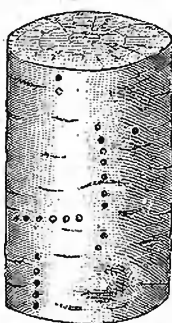
Рис. 1. Обрѣзокъ сучья березы, покрытой корою, на которой видны ряды отверстій, ведущихъ въ гнѣздо заболонника.
